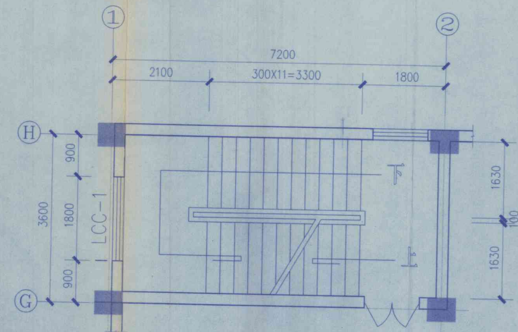
三、四层平面
