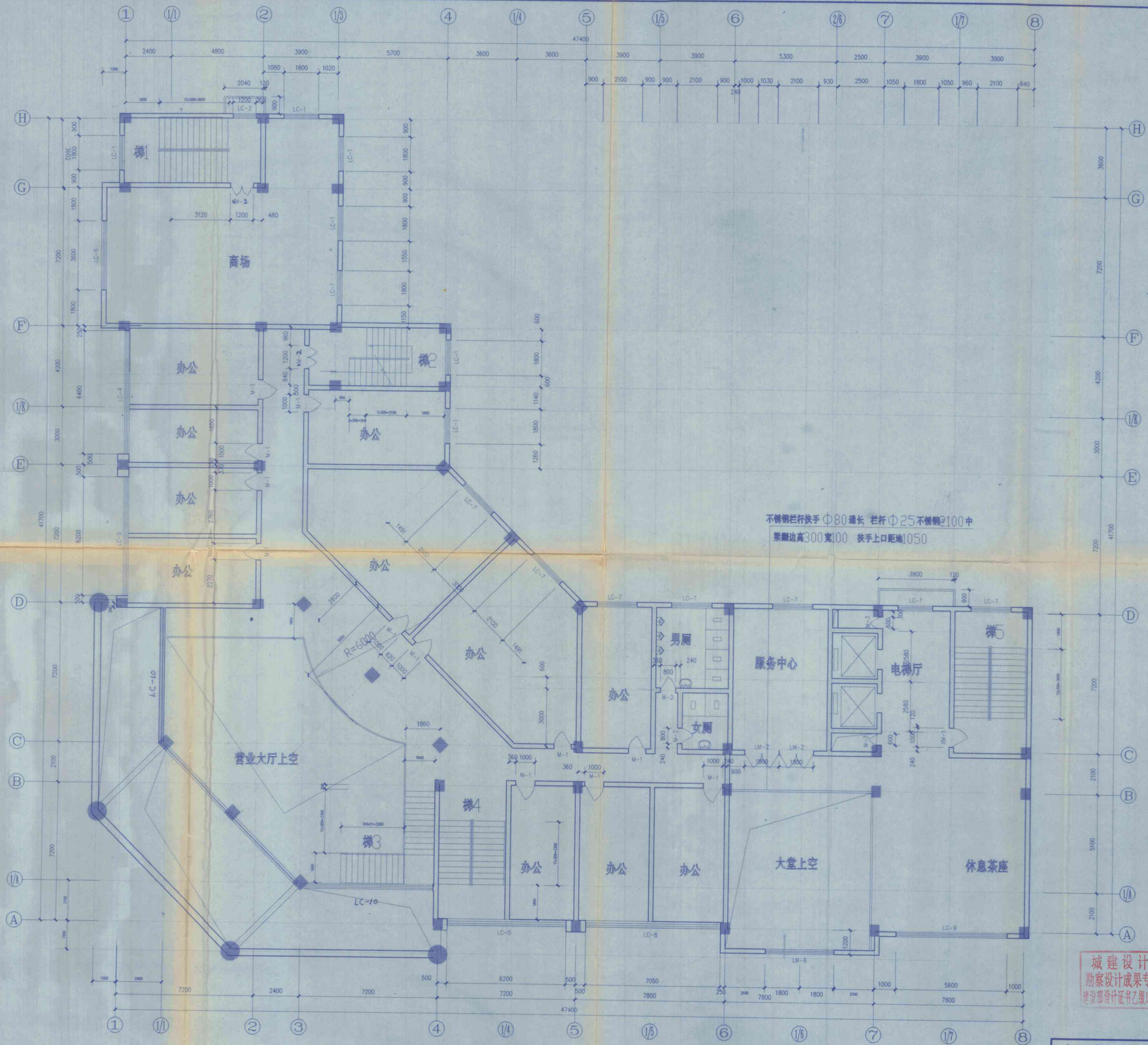
二层平面 1:100
