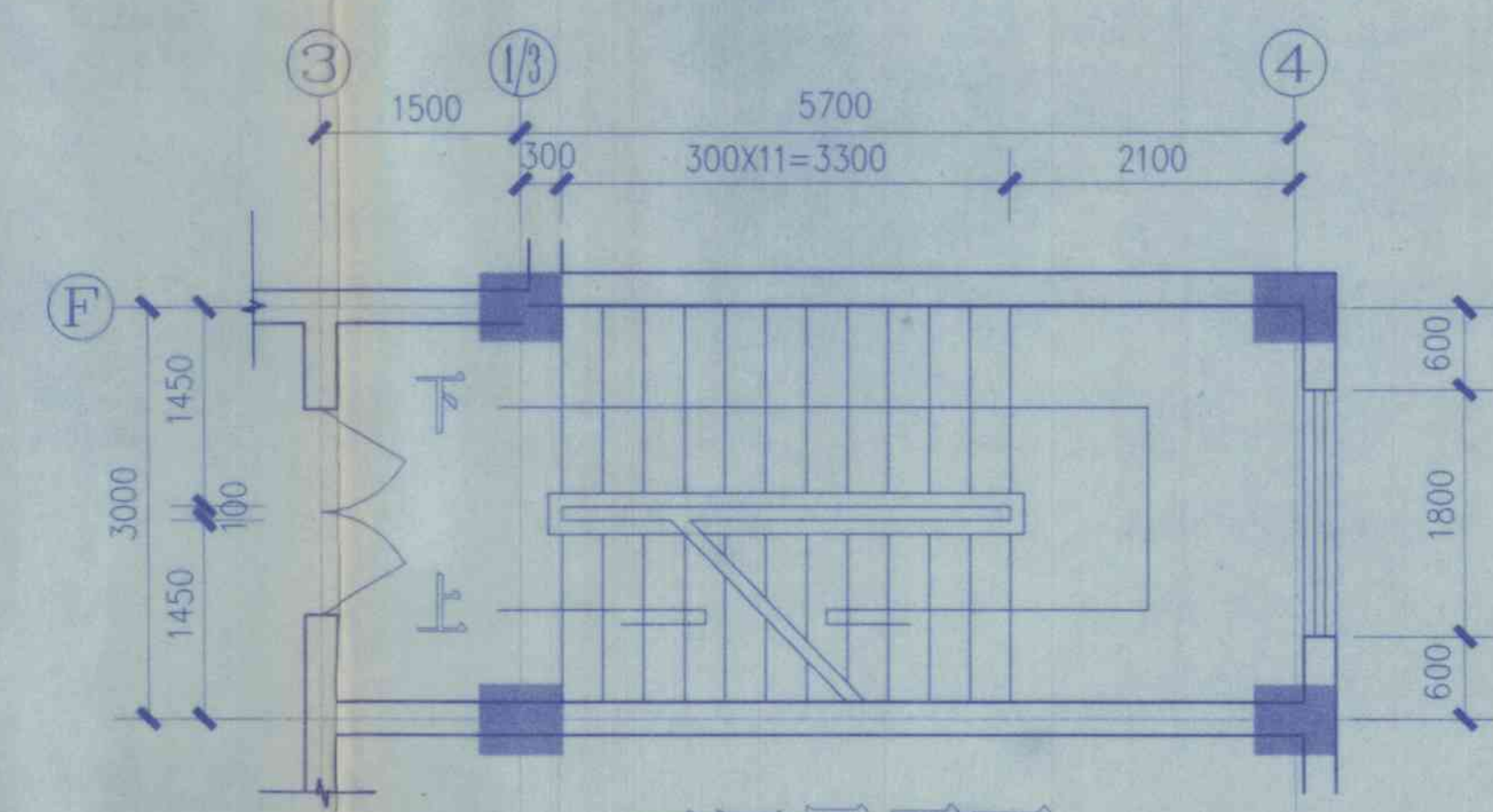
三、四层平面
