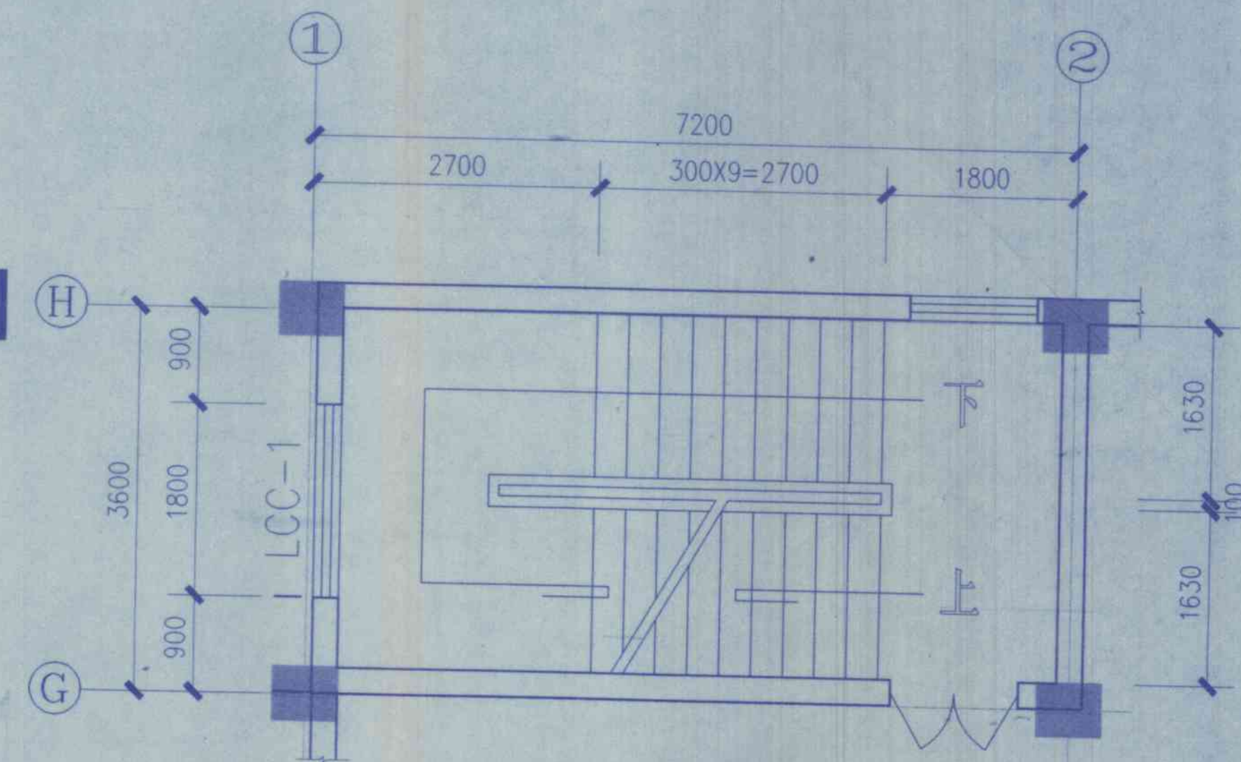
五、六层平面
