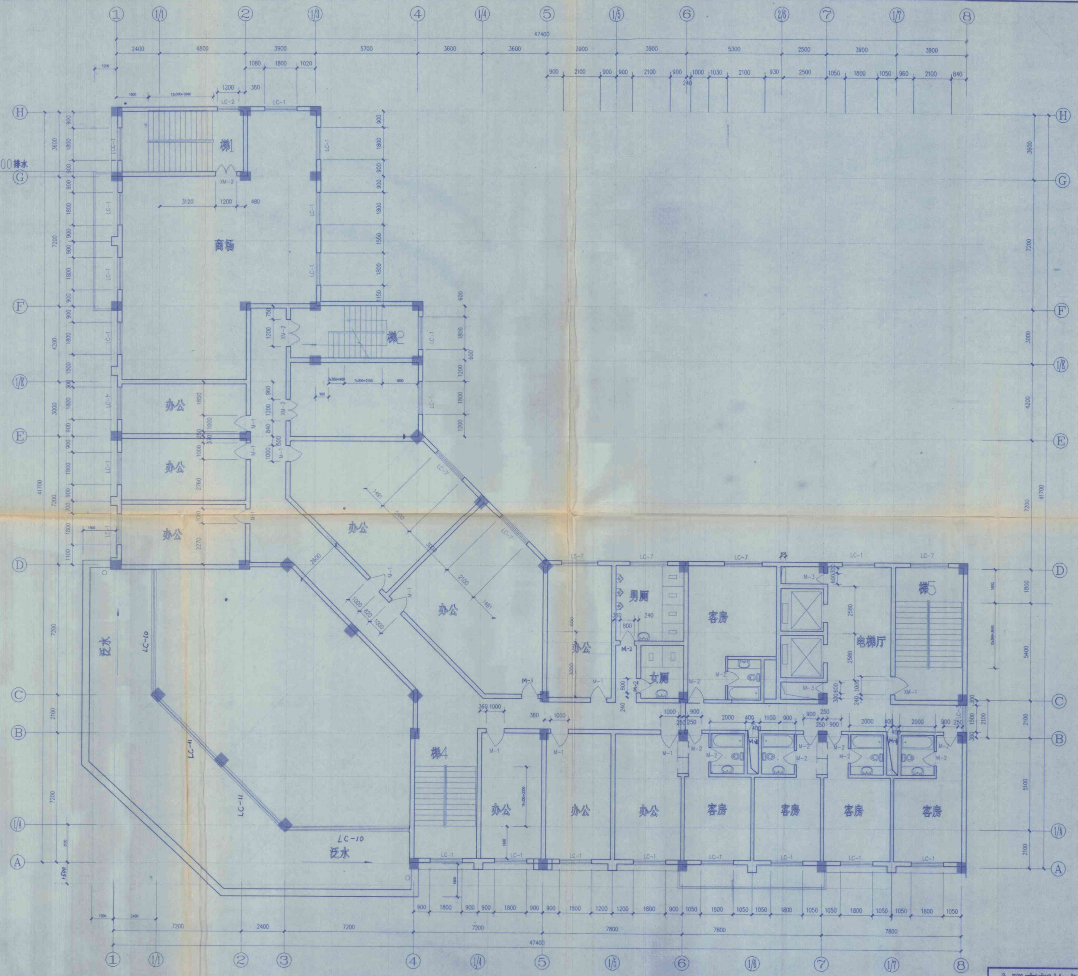
三层平面 1:100
