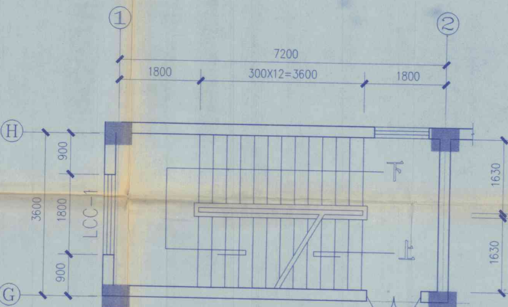
二层平面
