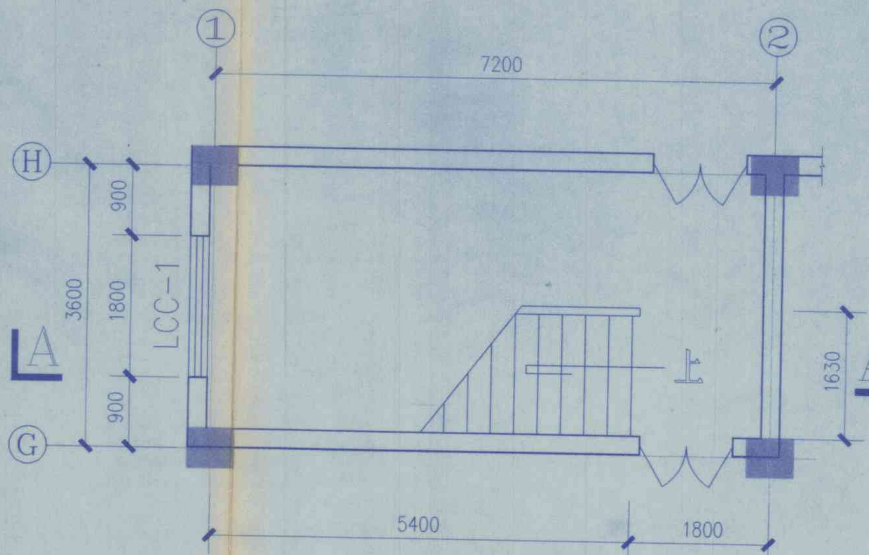
底层平面
