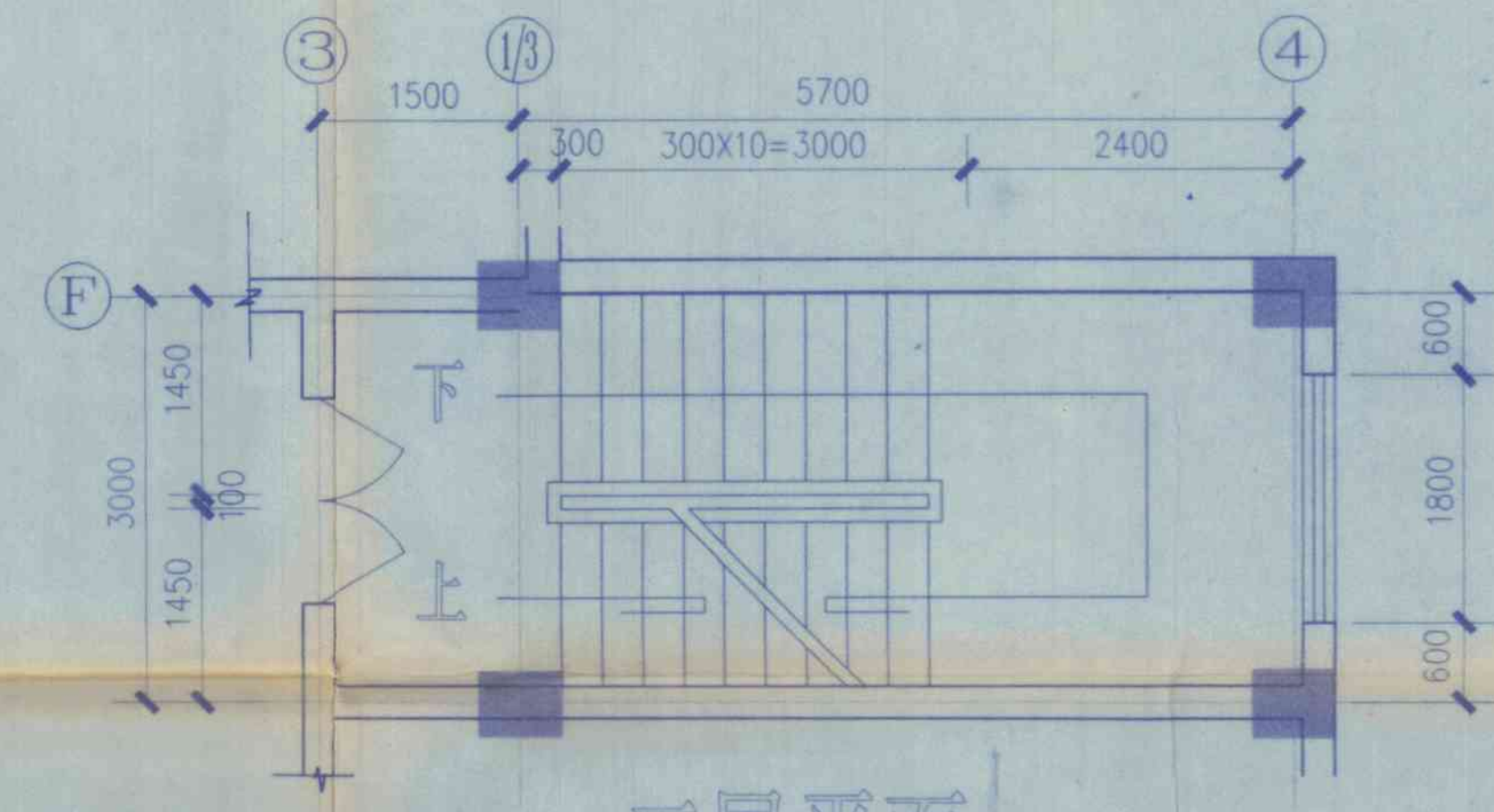
二层平面
