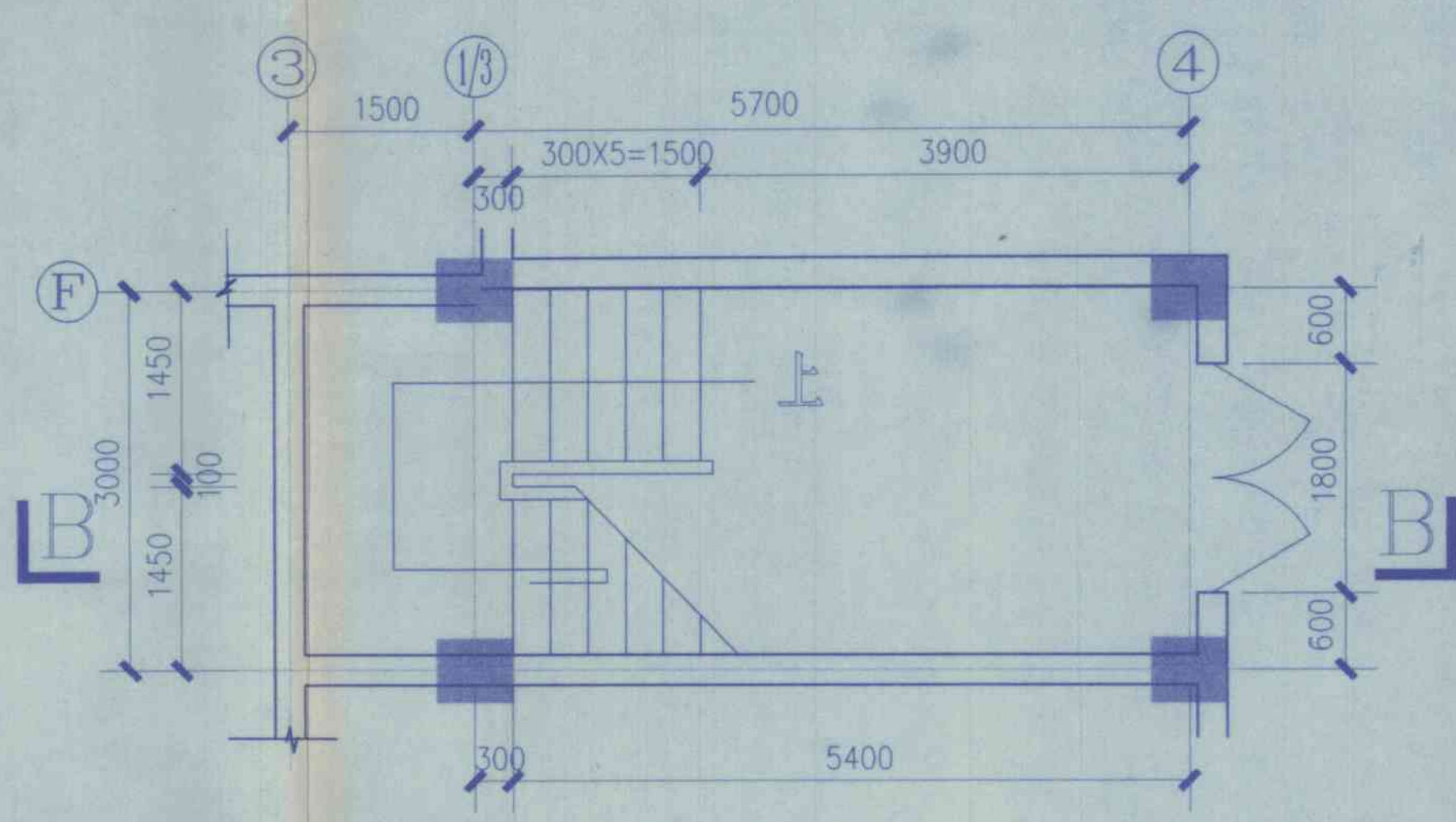
底层平面
