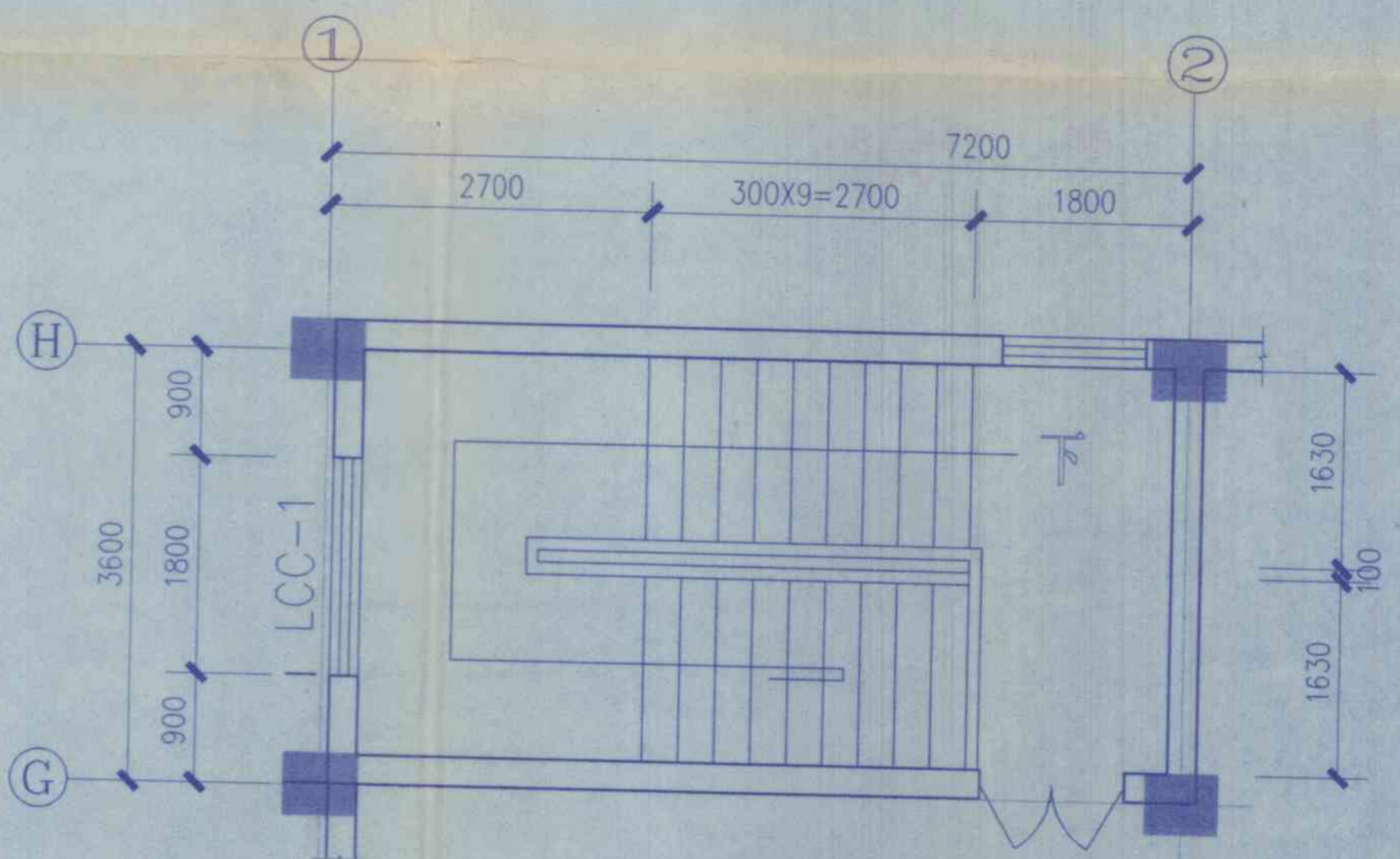
顶层平面
